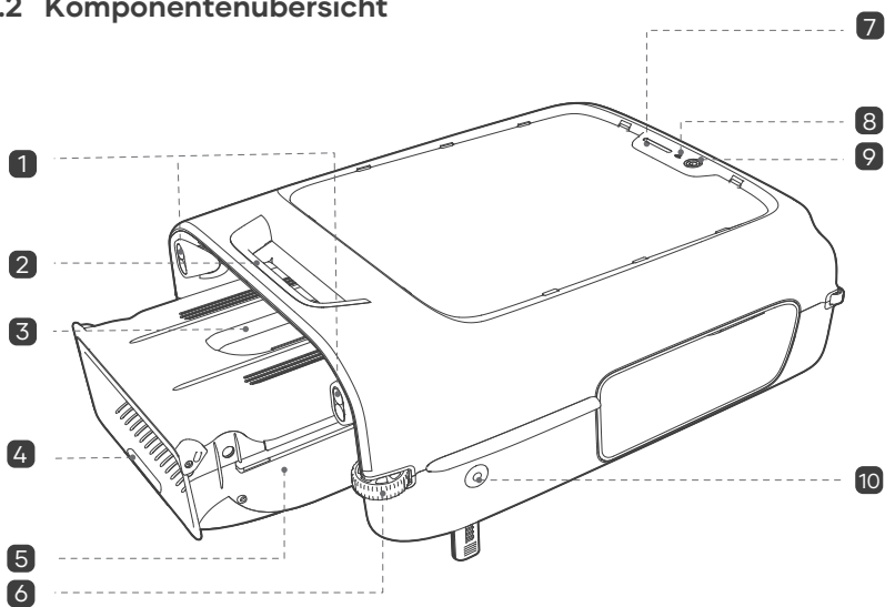
Reiniger (Seitenansicht)
